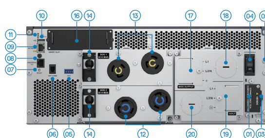
Smart-UPS Ultra 8、10kVA 背面
