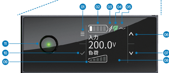
Smart-UPS Ultra 8、10kVA 前面
